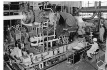
性能試験中のタイの製糖工場向け バイオマス発電用蒸気タービン
